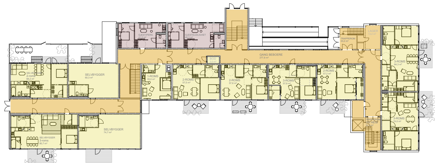
Øvre plan
